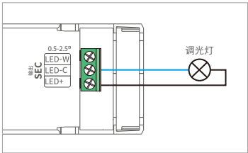
单路单通道—单路全功率输出
