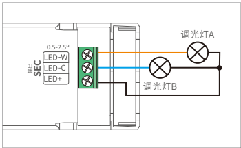
两路双通道—每路最大输出总功率50%
